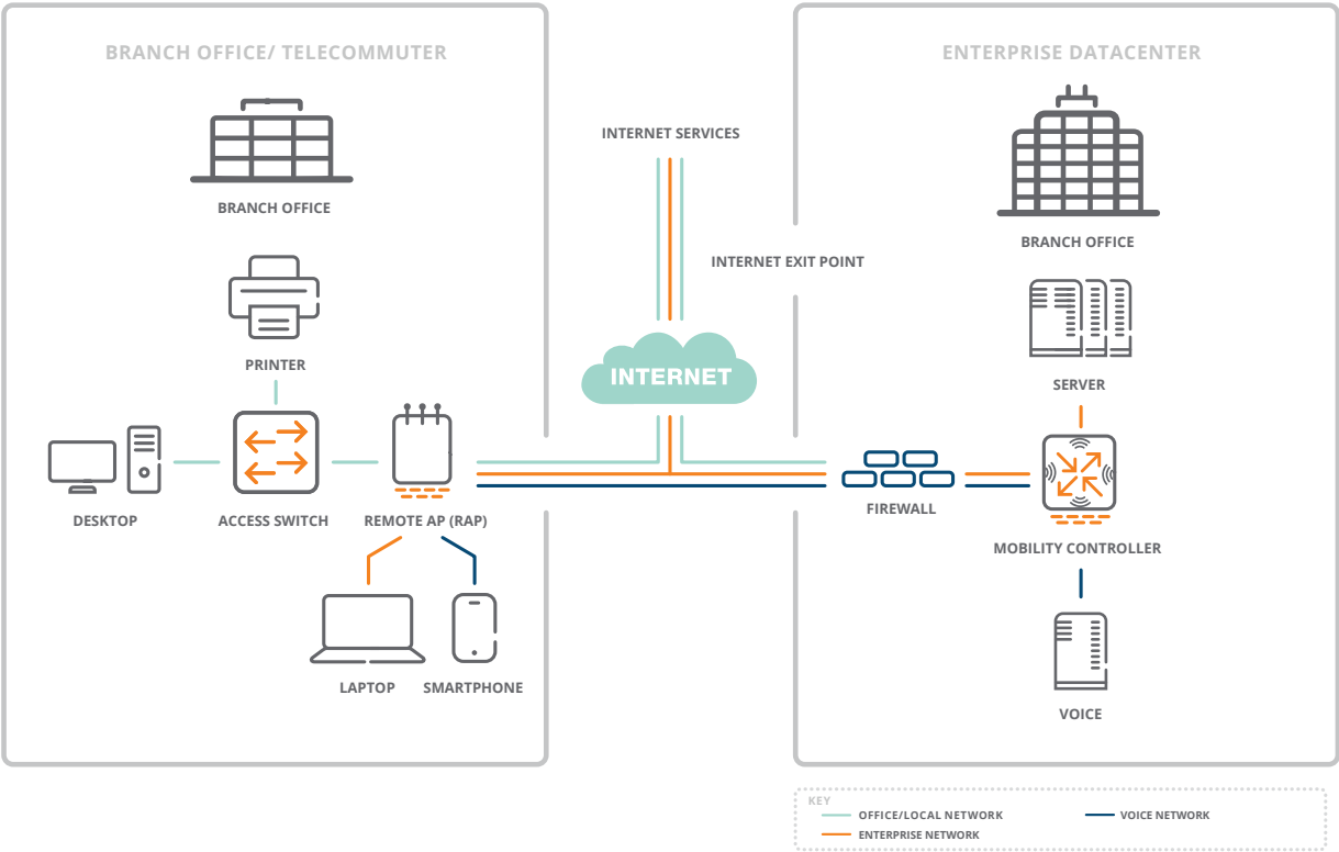
图3：与微型分支机构和小型办公场所建立安全移动连接的Aruba远程接入点
